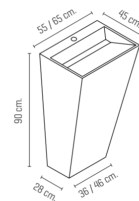
Detalle lavabo de pie OXFORD con orificio para grifería.
