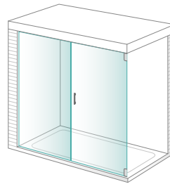
Ducha 1 fijo y 1 puerta pivotante en línea para combinar a 90°, a techo
