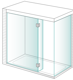
Ducha 3 fijos con escuadras, a techo
