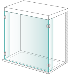
Ducha 3 fijos con escuadras, a techo
