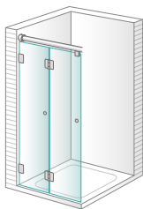
Ducha 2 puertas plegables en línea con bisagras a pared para combinar a 90°
