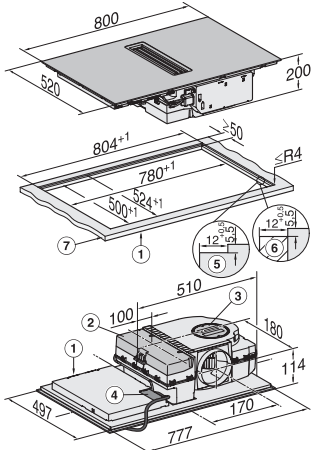
Instalación enrasada
