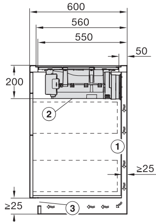
Recirculación Plug&Play
