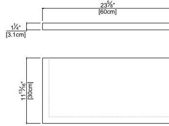
Technical Step Left Corner / Peldaño Técnico Esquina Izquierda / Nez de Marche Technique Coin Gauche
