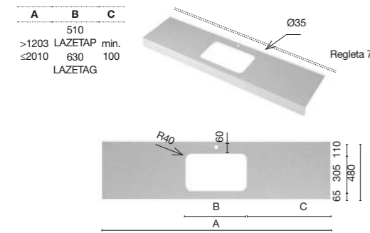
Encimera para lavabo bajoplano Zeta centrado
