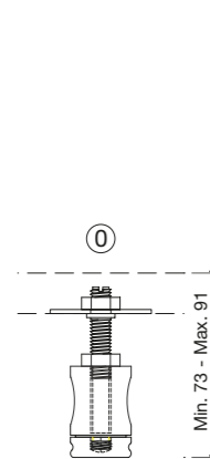
ESP-Altura mín. y máx. de SEP-system con el kit básico + 1 juego (sin plato)
