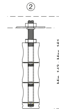
ESP-Altura mín. y máx. de SEP-system con el kit básico + 2 juegos (sin plato)
