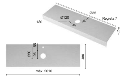
Encimera para lavabo sobremesa lota centrado
