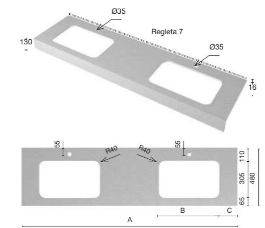
Encimera para 2 lavabos bajoplano Zeta
