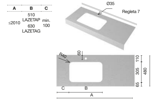
Encimera para lavabo bajoplano Zeta desplazado
