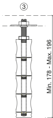
ESP-Altura mín. y máx. de SEP-system con el kit básico + 3 juegos (sin plato)
