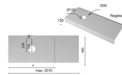
Encimera para lavabo sobremesa lota desplazado
