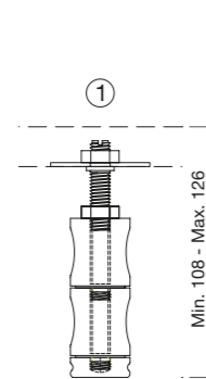
ESP-Altura mín. y máx. de SEP-system con el kit básico + 1 juego (sin plato)
