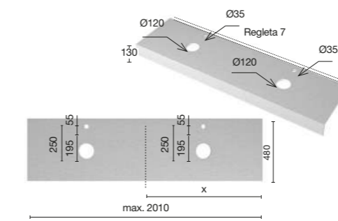
Encimera para lavabo sobremesa lota
