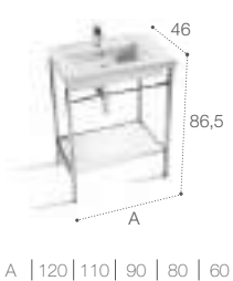
Estructura
